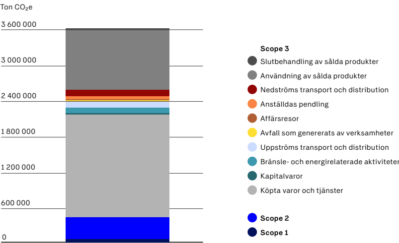
Beräknade utsläpp av växthusgaser (ton), basår 2019
