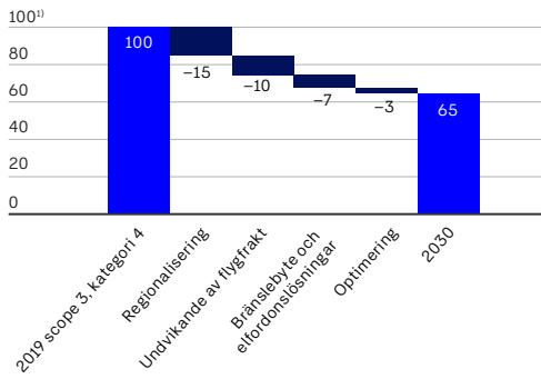
Relativt bidrag av strategiska hävstänger till uppnåendet av S3, C4 2030-målet
