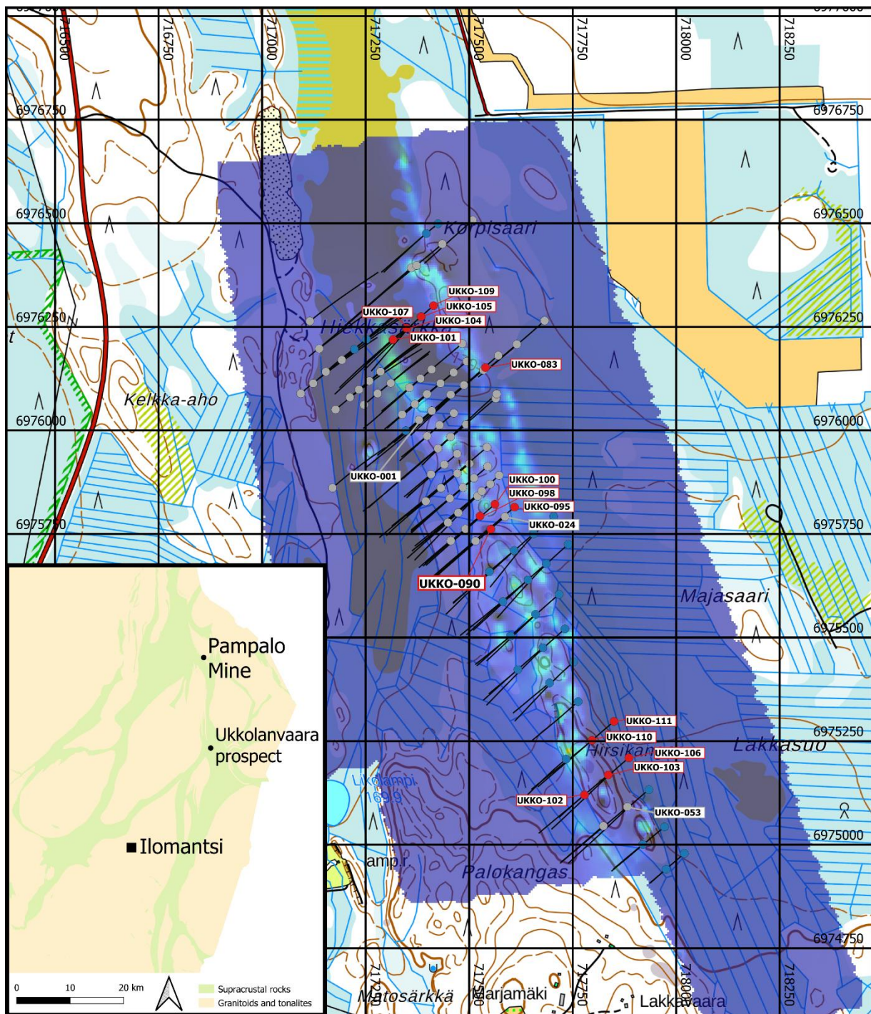
Kuva 1) Ukkolanvaaran 2026 kairareikien sijaintikartta, pohjana magneettinen totaali-intensiteettikartta
