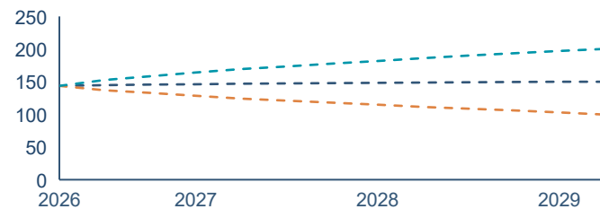
EUR / ISK
