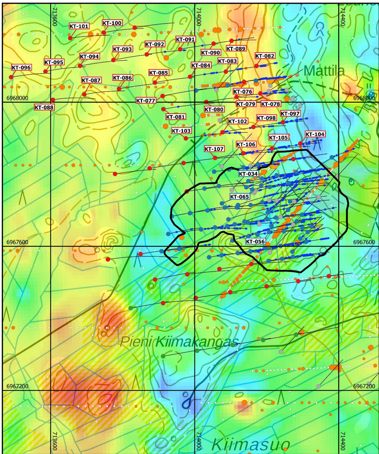
Figure 1 – Kuittilan kairareikien sijainnit kartalla, pohjana geofysikaalinen IP-varautuvuuskartta
