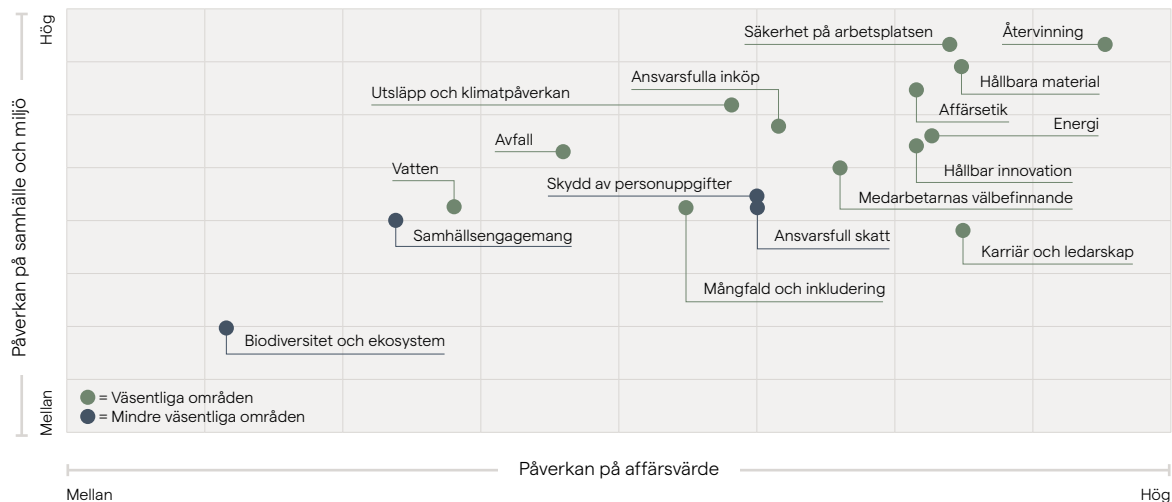
Gränges Väsentlighetsanalysmatris
